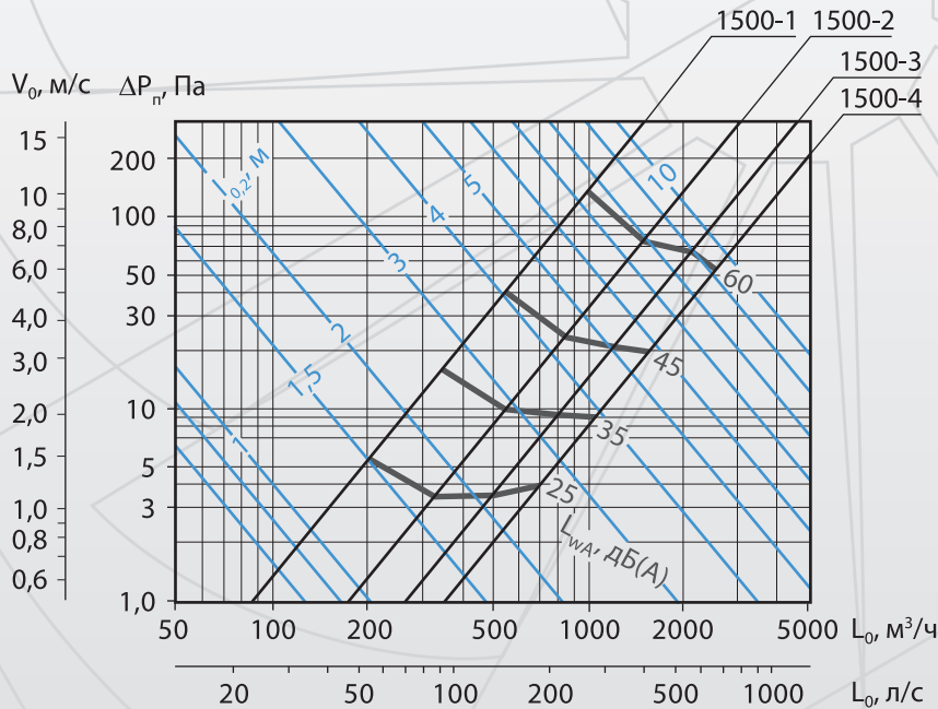
Аэродинамические и акустические характеристики воздухораспределителей ПВТ длиной 1500 мм при подаче воздуха в помещение по схеме 2 быстрозатухающим потоком перпендикулярно панели
