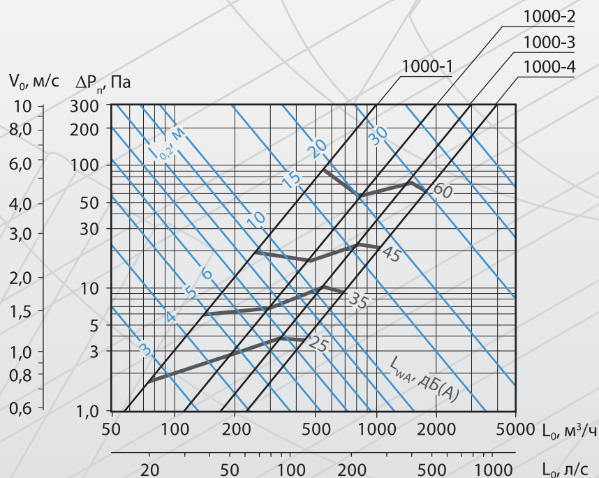
Аэродинамические и акустические характеристики воздухораспределителей ПВТ длиной 1000 мм при подаче воздуха в помещение по схеме 3 потоком, направленным в одну сторону в плоскости панели
