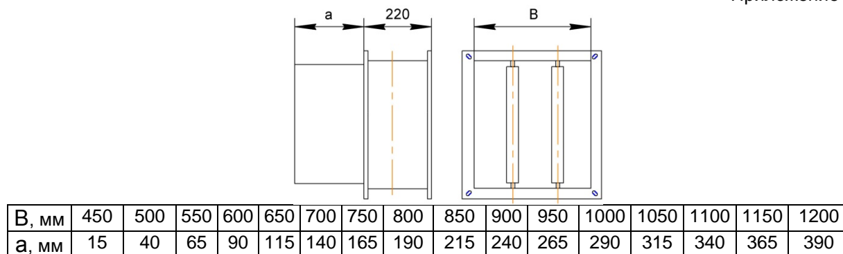
Рис.3. Размеры вылета заслонок в открытом положении за пределы клапана исполнений НО(К2)
